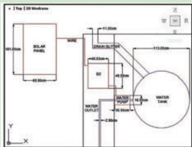
Gambar 4. Reka Bentuk prototaip menggunakan perisian AutoCAD.
